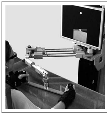
Figure 2.11 Braccio di Ferro. Reprinted with permission (www.iit.it).
